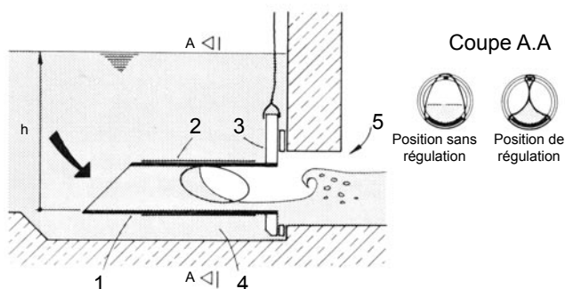
Fig. 2 : Régulateur à membrane UFT-FluidHose type I.
