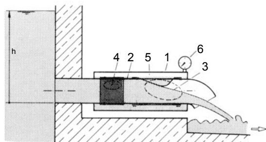
Fig. 3 : Régulateur à membrane UFT-FluidHose type U.
